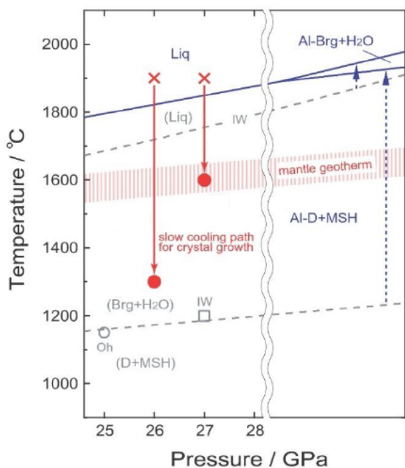
図2. 本研究で推察された \text{MgSiO}_3 系 (灰色の点線) と \text{Al}_2\text{O}_3 成分を含有した \text{MgSiO}_3 系 (青色の実線) の水の飽和条件下での可能な安定関係。D: D相, Brg: \text{MgSiO}_3 ブリッジマナイト, Al-D: Al-D相, Al-Brg: Al含有 \text{MgSiO}_3 ブリッジマナイト, Liq: 液相, MSH: 残存した \text{MgO-SiO}_2\text{-H}_2\text{O} 成分。( ) 付きと ( ) 無しの安定領域は、それぞれ \text{Al}_2\text{O}_3 成分を含有していない系と含有している系の領域を示している。IW (Ito & Weidner, Geophys. Res. Lett. 13, 464-466, 1986) および Oh (Ohtani et al., Phys. Chem. Miner. 27, 533-544, 2000) は文献から引用したデータである。赤色の×印、●印、↓印は、それぞれ本研究での高压結晶成長実験における最高保持温度、急冷温度、徐冷パスを示している。青色の長い点線矢印と短い点線矢印は、それぞれ D+MSH と Brg+H 2 O 間の相境界および液相線が \text{Al}_2\text{O}_3 成分を含有することによって高温側へ移動することを示している。
